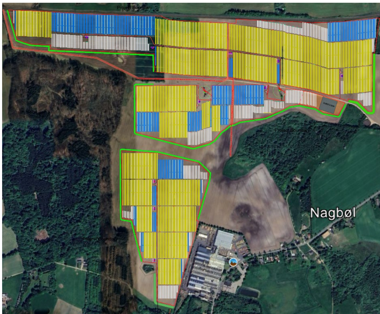
Figur 1 - Oversigtskort over Solcelleanlæg Nagbøl. Den grå firkant angiver placeringen af BESS-anlægget.
