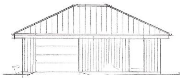
Facade syd 1:100
