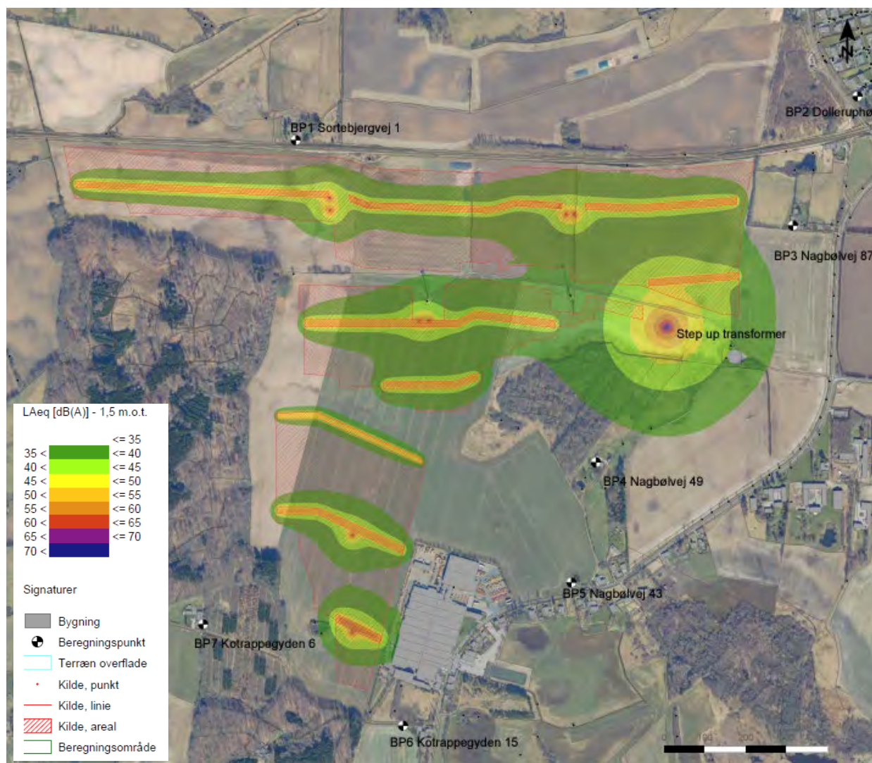
Figur 6-2 Støjdbredelseskort - natperiode.
