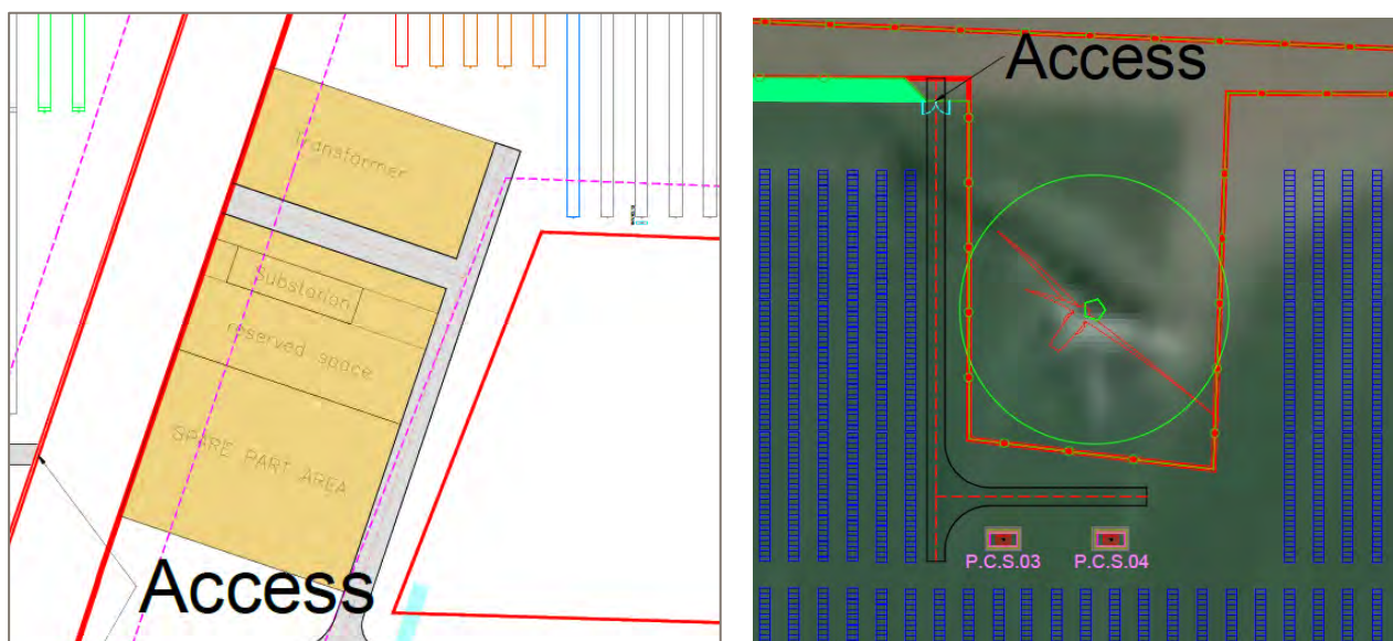
Figur 11-1 T.v.: Udsnit af projektskitse for teknikområde for power-transformer (eksempel fra andet, tilsvarende Ænergy projekt). Se endvidere eksempelfoto Fig 1-6 og projektbeskrivelsen. T.h.: Udsnit af projektskitse for areal omkring MV-station syd for den ene vindmølle ved Nagbøl. Hver MV-station har en størrelse på ca. 4 x 6 m.
