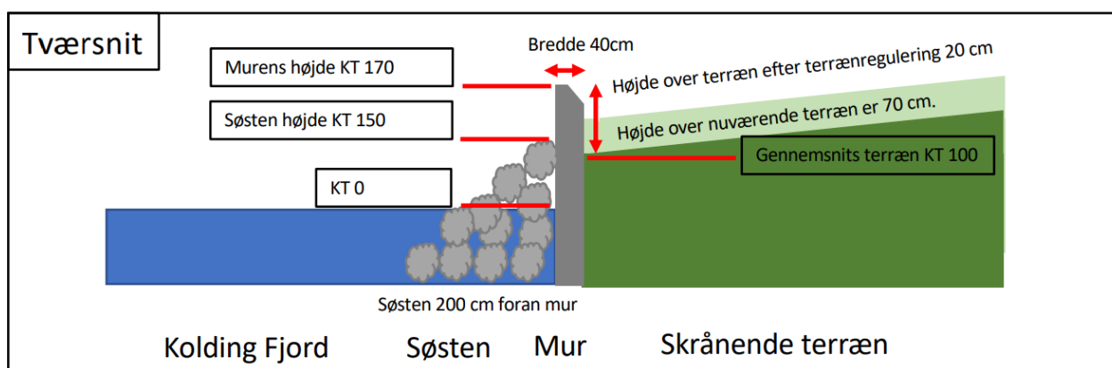
Figur 2. Snittegning, der viser dimensionerne på betonmur med stenkastning foran. Terrænregulering med 0,5 m på grunden bag muren er ikke en del af denne tilladelse.
