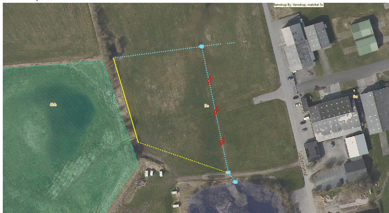
Figur 2: Den lyseblå stiplede linje angiver den omtrentlige placering af eksisterende, ældre drænrør. De røde streger markerer det dræn der ikke længere fungerer. Den gule stiplede linje angiver den omtrentlige placering af den nye drænelledning og den gule streger angiver den omtrentlige placering af det faste rør.
