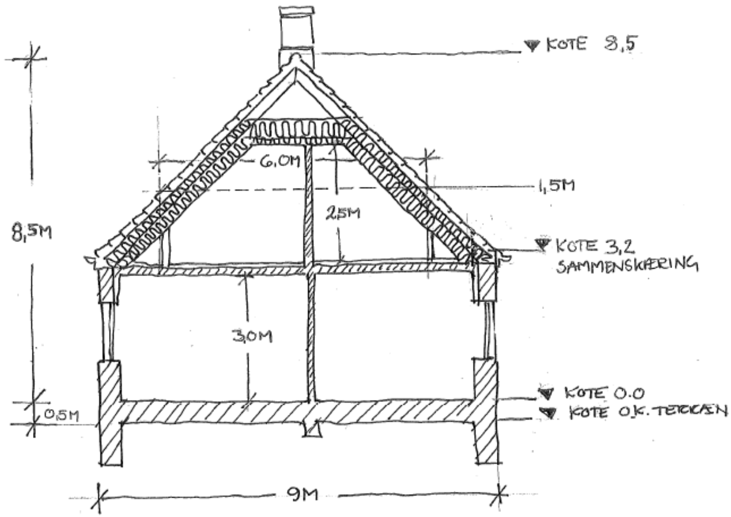
SNIT 1:50
